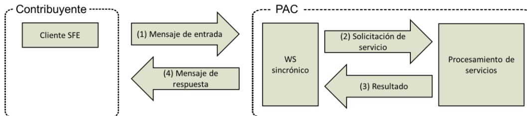
Ilustración 5 – Servicio Web Sincrónico
